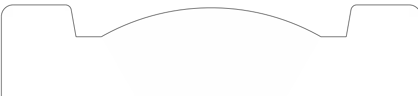
1552 Rosette 1.000" x 4.500"
