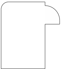
1809 Backband 1.125" x 1.000"
