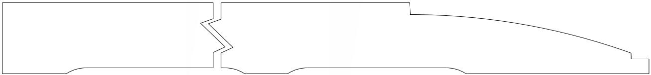
3680 Base 0.750" x 8.000"
