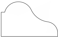
3076 Base cap 0.625" x 1.000"
