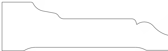
IO54 Casing 0.875" x 3.000"
