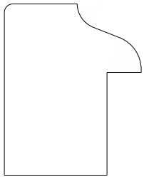
1040 Backband 1.250" x 1.000"
