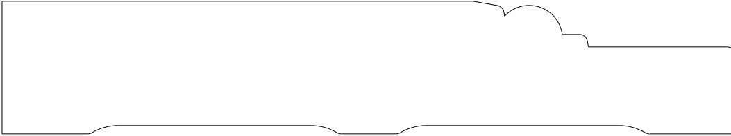
3548 Base 1.000" x 5.500"
