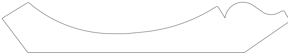
2558 Crown 0.875" x 5.000"
