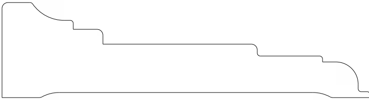
1539 Casing 1.000" x 3.875"
