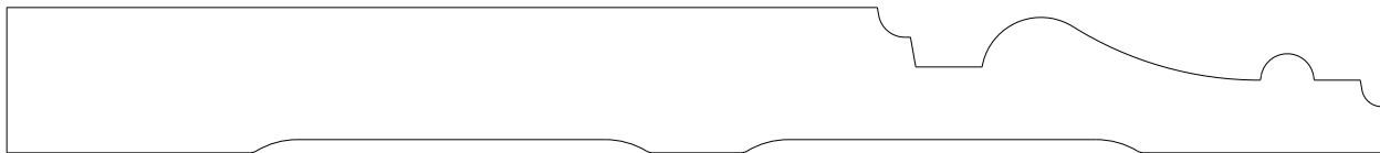
3036 Base 0.687" x 6.500"
