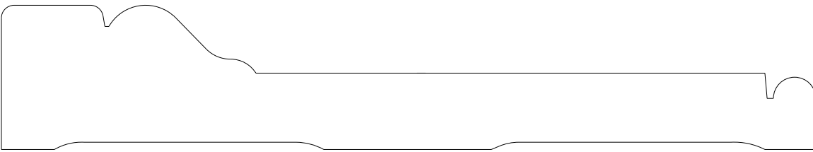
IO32 Casing 1.000" x 6.000"
