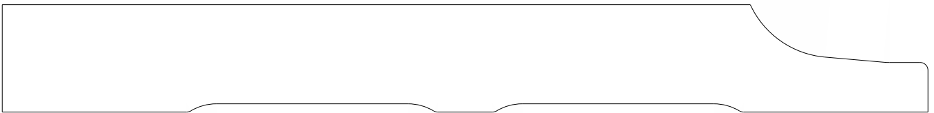
3550 Base 0.812" x 7.000"
