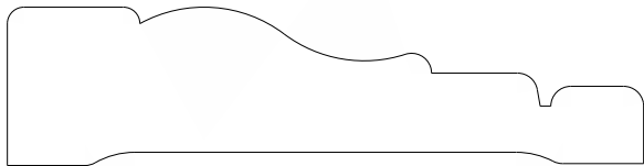
IO29 Casing 0.750" x 3.000"
