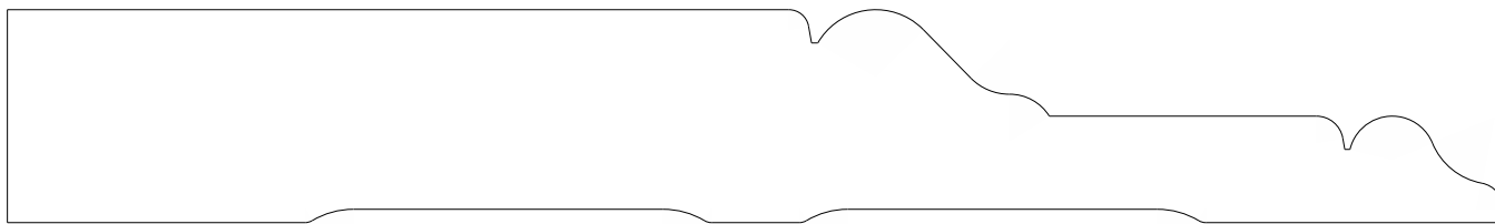
3038 Base 1.000" x 7.000"
