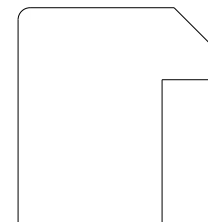
1310 Backband 1.125" x 1.000"
